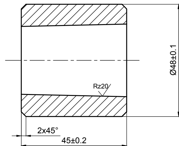
BẠC CÔN
