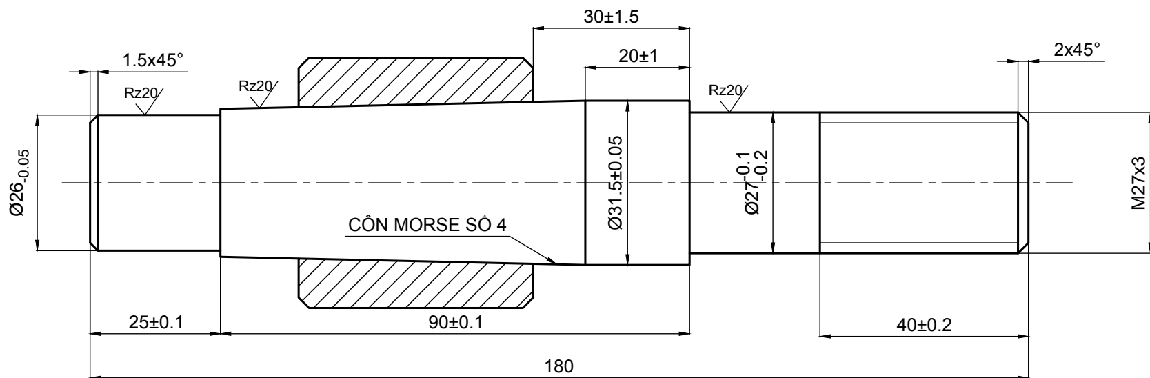
TRỤC CÔN
